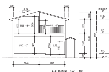
A-A' 断面図 S=1:100
