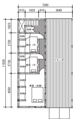
2階平面図 S=1:100
