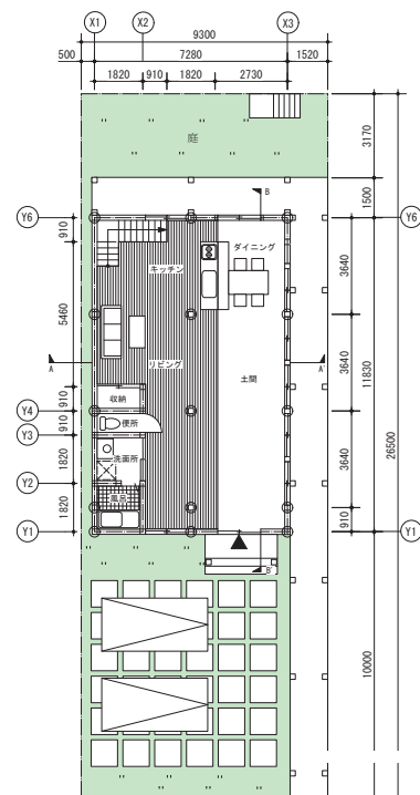
配置図兼1階平面図 S=1:100
