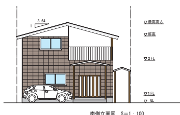
南側立面図 S=1:100
