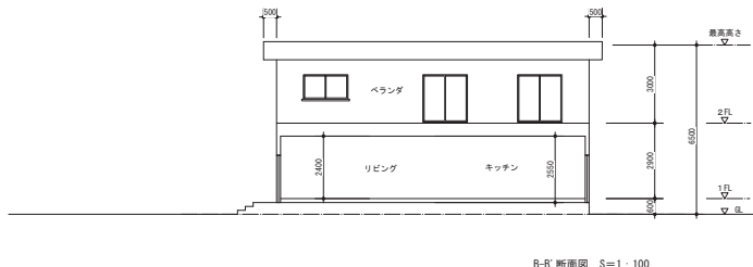
B-B' 断面図 S=1:100
