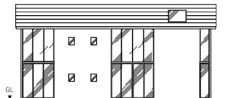
東側 立面図 S=1:100
