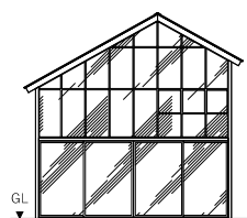
南側 立面図 S=1:100
