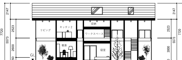
A-A'断面図 S=1:100
