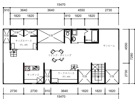
2階平面図 S=1:100
