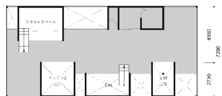
3階平面図 S=1:100
