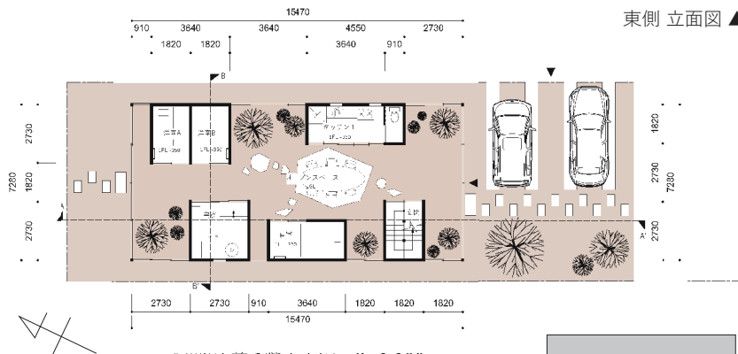
配置図 兼 1階平面図 S=1:100
