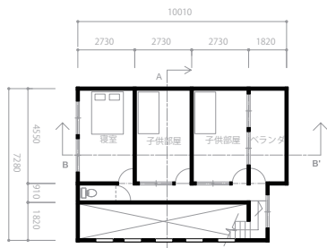
2 階平面図 S=1:100
